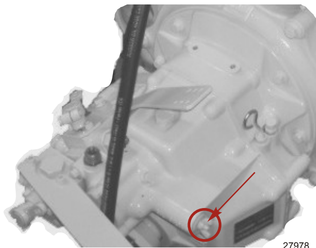
Befestigungsmutter des Getriebeölfilters
