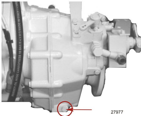
Getriebeöl-Ablassschraube
